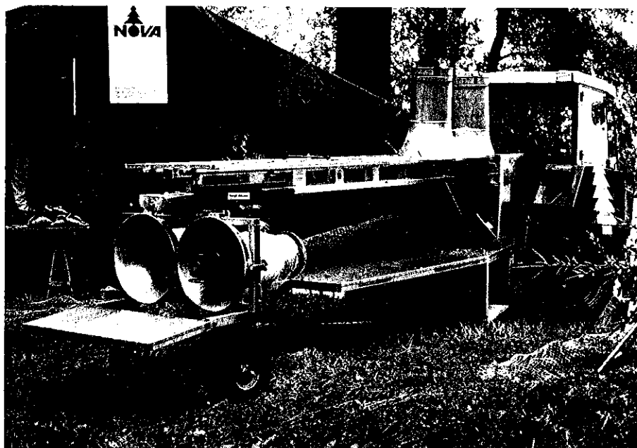
EVA III netmaskine. Bemærk tragtene der står oven på maskinen. Man ser tydeligt den runde overgang fra konus til cylinder.
