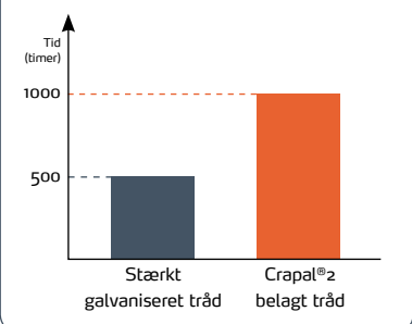
Salttågetest
